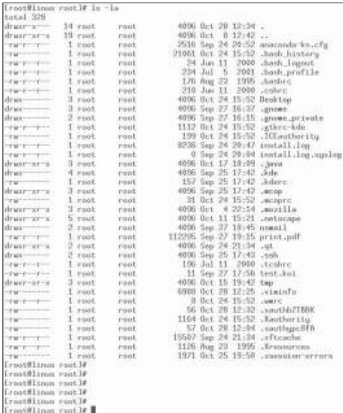
Файловая система UNIX.
