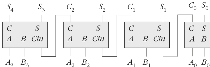
Последовательный сумматор.
